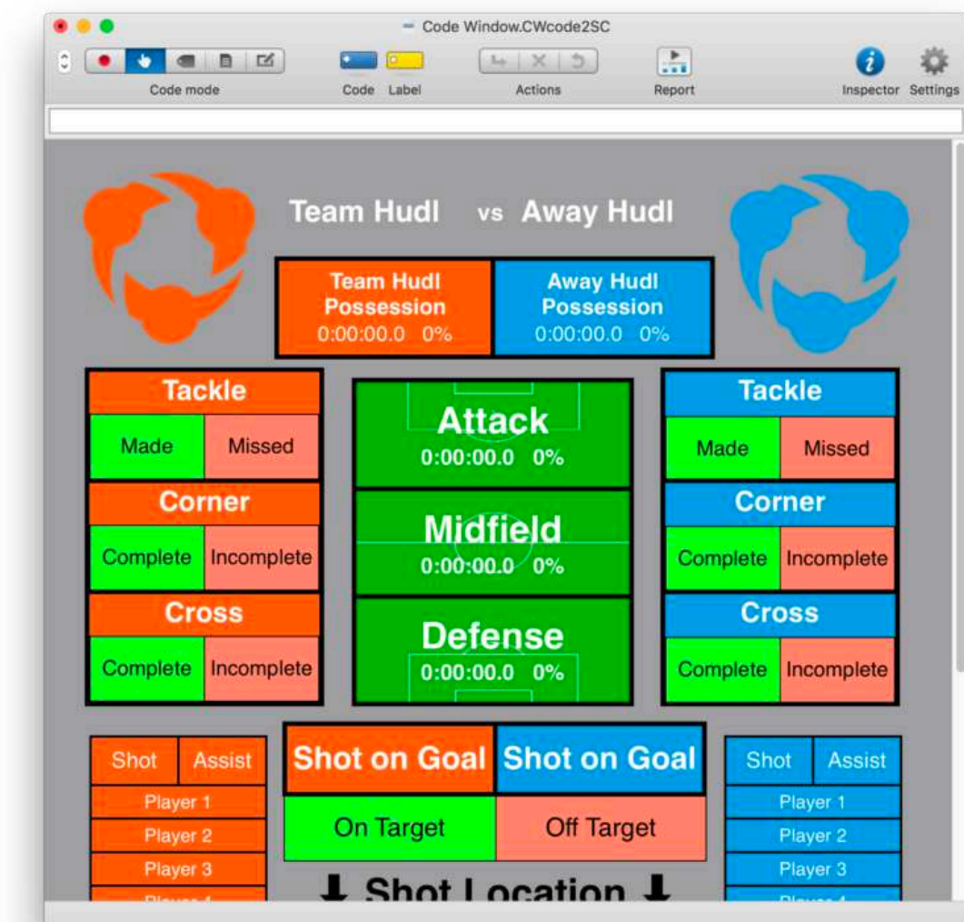
Logiciel ?
